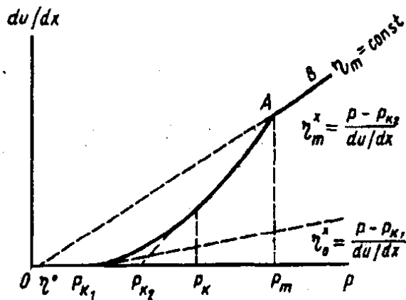
Рис. 1. Реологічна крива, або крива течії в системі координат «напряга (P) зсуву – градієнт швидкості (du/dx) деформації»
