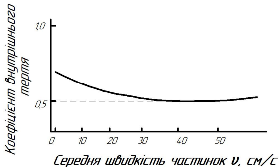
Рис. 2. Залежність коефіцієнта внутрішнього тертя віброваної маси від середньої швидкості переміщення частинок, см/с : v = A2f , де A – амплітуда коливань; f – частота коливань, Гц
