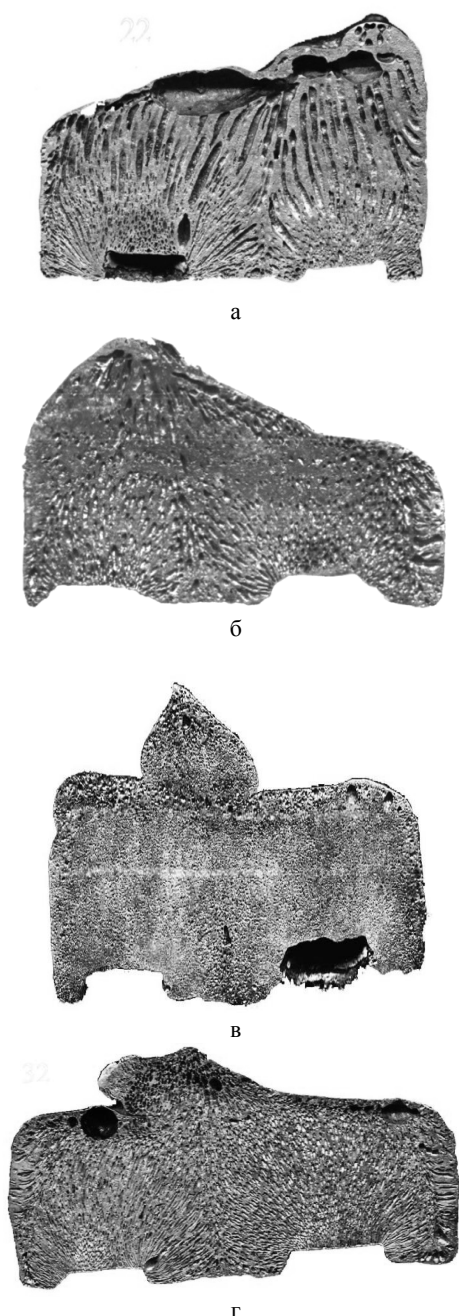
Рис.2. Виды структур отливок медных газаров полученных при различных параметрах плавки: а – R_{нас.} = 0,2\text{МПа} , R_{кр.} = 0,05\text{МПа} ; б - R_{нас.} = 0,25\text{МПа} , R_{кр.} = 0,1\text{МПа} ; в - R_{нас.} = 0,3\text{МПа} , R_{кр.} = 0,25\text{МПа} ; г - R_{нас.} = 0,3\text{МПа} , R_{кр.} = 0,15\text{МПа} / Types of structures of copper castings Gazarov obtained by melting various parameters: а - R_{нас.} = 0,2\text{МПа} , R_{кр.} = 0,05\text{МПа} ; б - R_{нас.} = 0,25\text{МПа} , R_{кр.} = 0,1\text{МПа} ; в - R_{нас.} = 0,3\text{МПа} , R_{кр.} = 0,25\text{МПа} ; г - R_{нас.} = 0,3\text{МПа} , R_{кр.} = 0,15\text{МПа}
