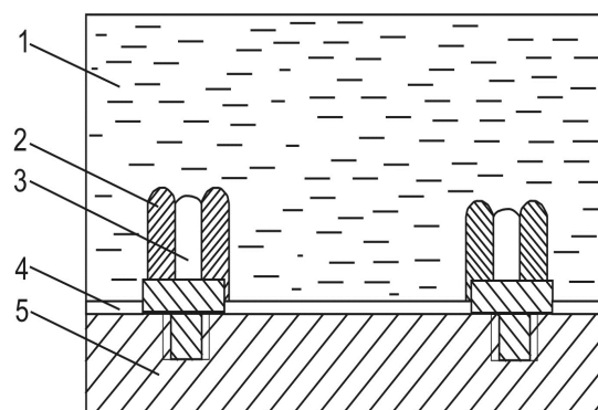
Рис. 1. Схема кристаллизации при взаимодействии двух параллельных аксиальных фронтов кристаллизации газара: 1 – расплав; 2 – металл; 3 – поры; 4 – противопожарное покрытие; 5 – холодильник кристаллизатора.
