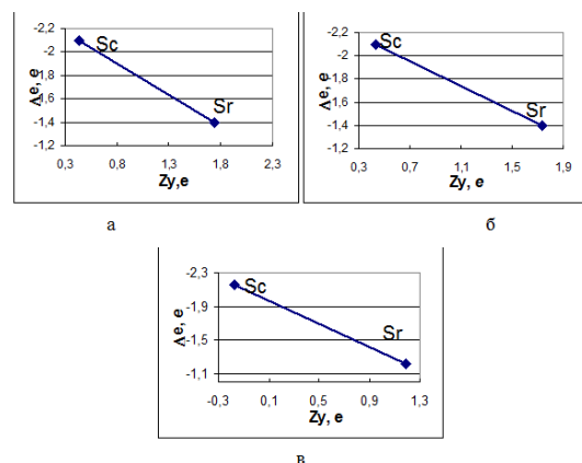
Рис. 1. Изменение степени направленности \Delta_e парных связей Si-X (а, б) и O-X (в) в сплаве АК7ч Al-Si-Mg-Fe (а) и Al-Si-Mg-Fe-O (б, в), где X – Sr и Sc/ The change in the degree of directionality of the \Delta_e pair bonds Si-X (а, б) and OX (c) in the alloy АК7ch Al-Si-Mg-Fe (а) and Al-Si-Mg-Fe-O (б, в), where X - Sr and Sc
