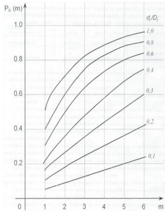
Рис. 2 – Залежність P_b(m) від m -ої кількості шкідливих факторів та d_j/D_j ( t_j^b t_j^p = \text{const} ) / Reliance P_b(m) from t -th number of harmful factors and d_j/D_j ( t_j^b t_j^p = \text{const} )
