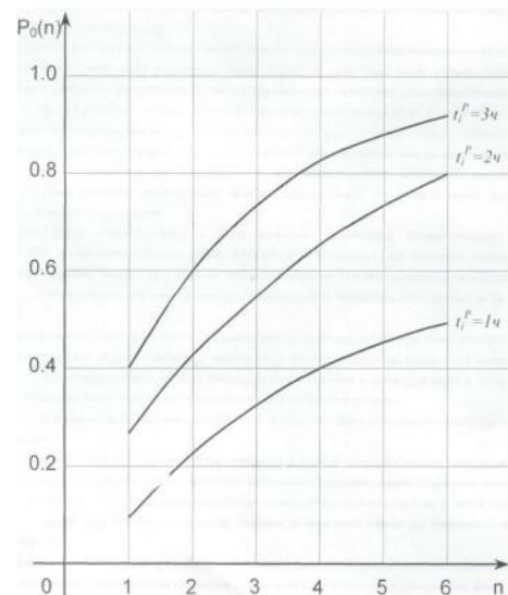
Рис. 1 – Залежність P_0(n) дії i -ої чисельності шкідливих факторів при t_j^p = \text{const} /
