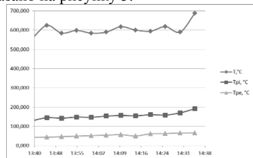
Рис.3. Графік зміни температур у процесі нагрівання Graphoftemperature redistribution
