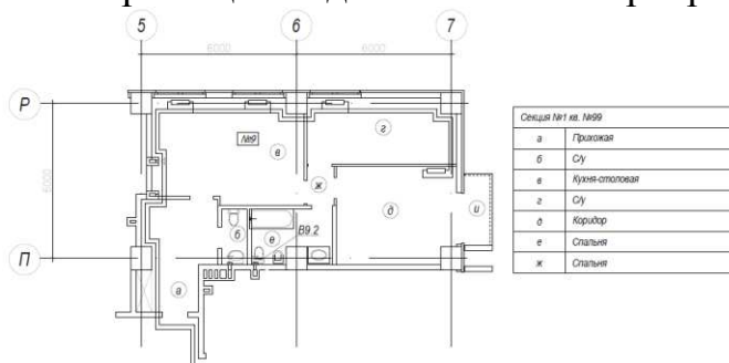
Рис. 5.32 Схема приміщення трьохкімнатної квартири та точки виміру.
