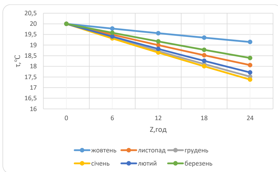
Рис.5.21 Залежності зміни значення очікуваної температури внутрішнього повітря t_b(Z) для середнього приміщення із зовнішніми огорожувальними конструкціями III типу, якщо вплив зовнішнього середовища на будівлі враховує дію сонячної радіації для випадку щільної забудови
