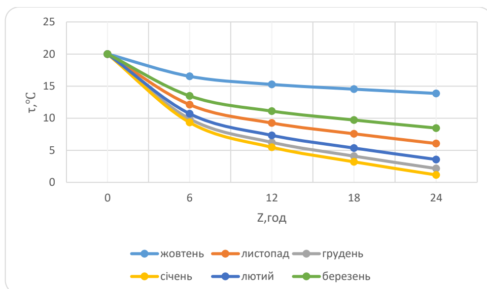
Рис. 4.24 Графік динаміки охолодження внутрішніх поверхонь приміщень при аварійному відключенні системи тепlopостачання на прикладі стіни V типу
