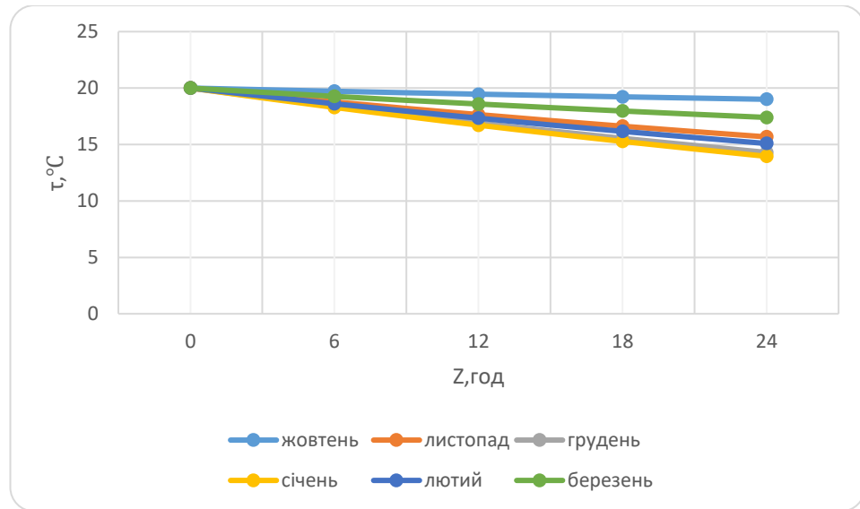
Рис.5.13 Залежності зміни значення очікуваної температури внутрішнього повітря t_v(Z) для середнього приміщення із зовнішніми огорожувальними конструкціями I типу, якщо вплив зовнішнього середовища на будівлі враховує дію сонячної радіації для випадку вільної розімкненої забудови
