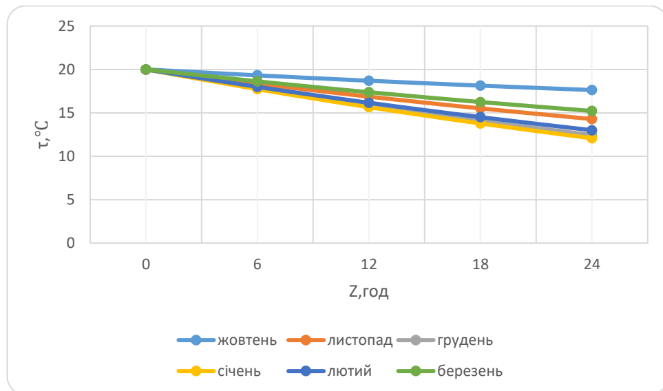
Рис.5.8 Залежності зміни значення очікуваної температури внутрішнього повітря t_b(Z) для середнього приміщення із зовнішніми огорожувальними конструкціями II типу, якщо вплив зовнішнього середовища на будівлі враховує дію сонячної радіації та вітру для випадку щільної забудови
