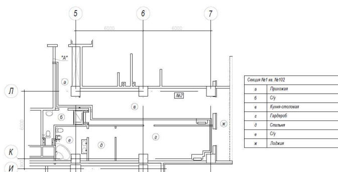
Рис. 5.31 Схема приміщення двокімнатної квартири та точки виміру.
