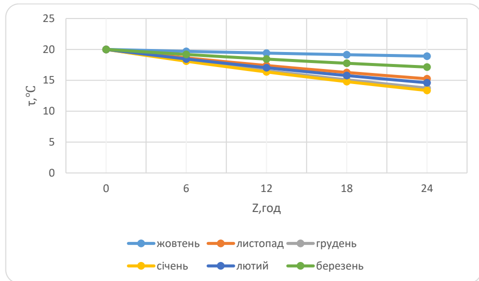
Рис.5.14 Залежності зміни значення очікуваної температури внутрішнього повітря t_b(Z) для середнього приміщення із зовнішніми огорожувальними конструкціями II типу, якщо вплив зовнішнього середовища на будівлі враховує дію сонячної радіації для випадку вільної розімкненої забудови
