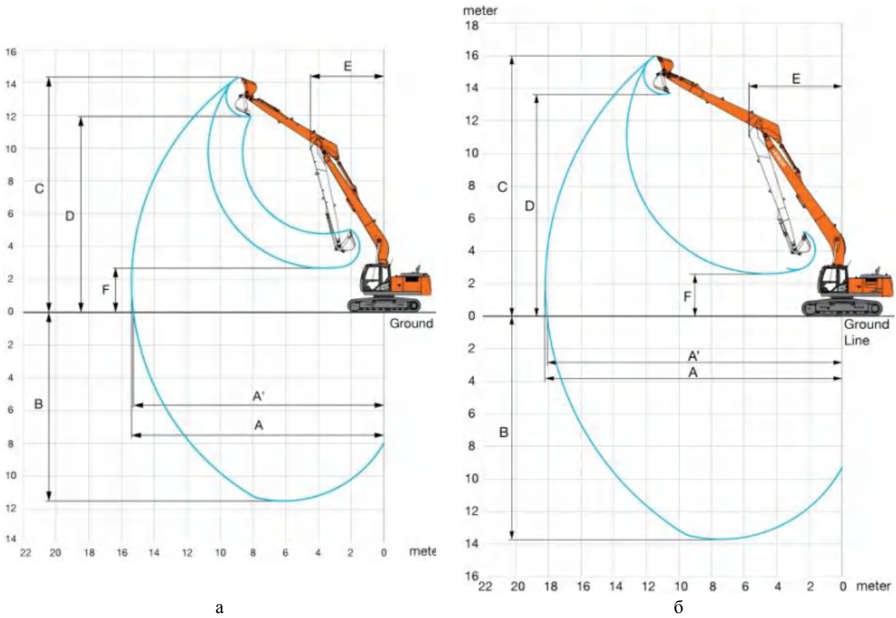
Рис. 2. Екксаватору фірми Hitachi: а – ZX 210LC; б – ZX 290LC.
