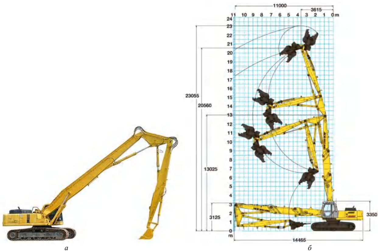
Рис. 5. Нові структури РО ОГЕ: а – экскаватор з трисекційним РО фірми ОЕМ; б – экскаватор Е 385LC фірми New Holland з багатосекційним РО змінної геометрії..
