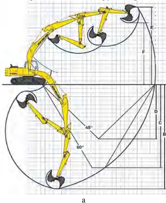
Рис. 4. Нові структури РО ОГЕ: а – екскаватор E215 BLC-M з трьома рукоятями фірми New Holland ; б – екскаватор PC240LC-10 фірми Komatsu зі збільшеними розмірами елементів РО.
