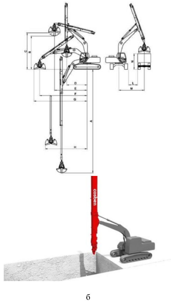
Рис. 9. Екскаратори з телескопічними рукоятями: а – Hitachi ZX210LC-5B; б – Cosben TA.
