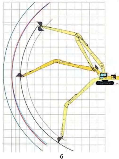
Рис. 4. Нові структури РО ОГЕ: а – екскаватор E215 BLC-M з трьома рукоятями фірми New Holland ; б – екскаватор PC240LC-10 фірми Komatsu зі збільшеними розмірами елементів РО.
