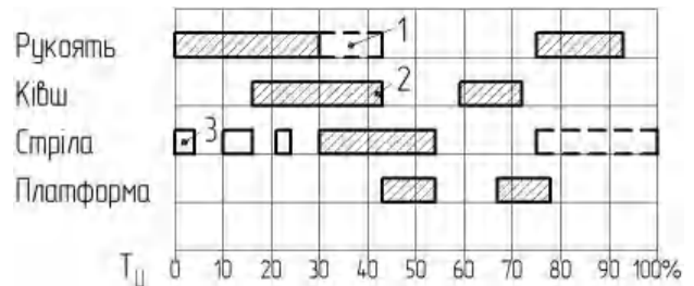
Рис. 10. Робочий цикл (циклограма роботи) екскаватора з обладнанням «зворотна лопата»: 1 – операції, виконання яких не потребує енергетичних затрат; 2 – операції, які потребують затрати енергії; 3 – короткострокові включення.
