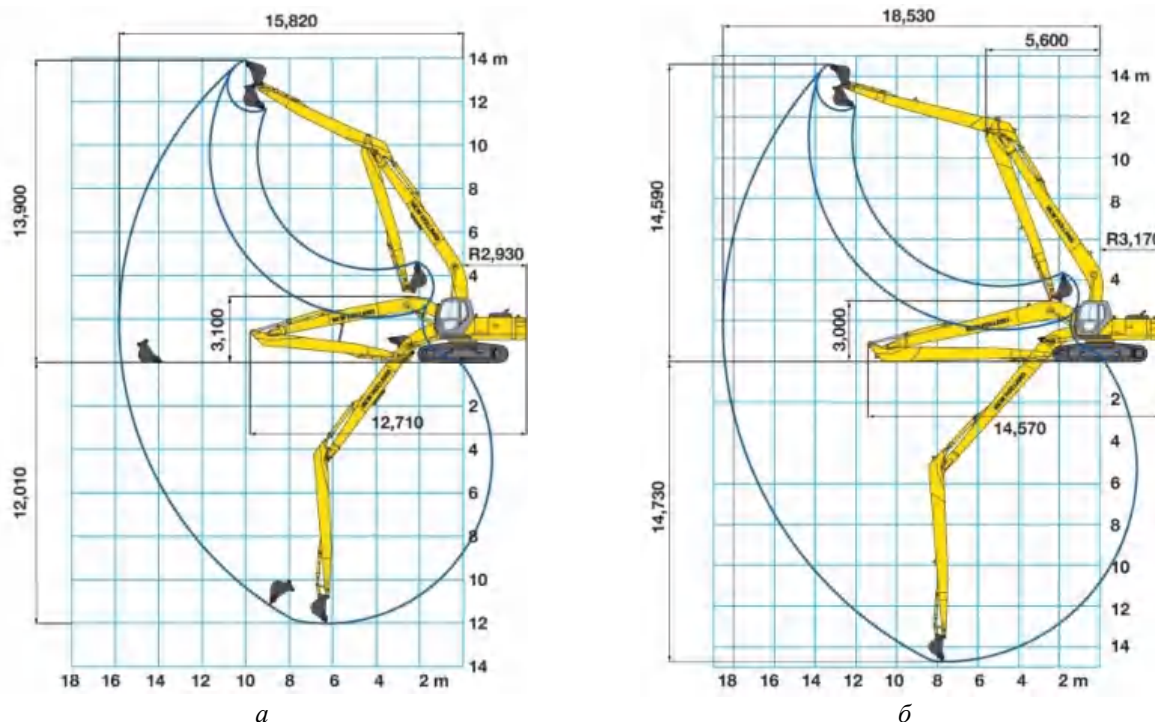
Рис. 1. Екскаватори фірми New Holland зі збільшеними розмірами РО: а – E 215 LC; б – E 265 LC.
