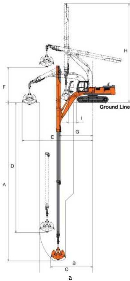
Рис. 9. Екскаратори з телескопічними рукоятями: а – Hitachi ZX210LC-5B; б – Cosben TA.
