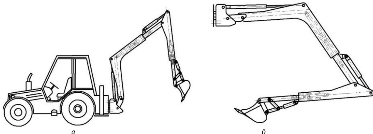
Рис. 12. Конструкція екскаватора з телескопічною стрілою та рукояттю по а.с. України №65783: а – загальний вигляд; б – телескопічне робоче обладнання при втягнутих телескопах стріли та рукояті.
