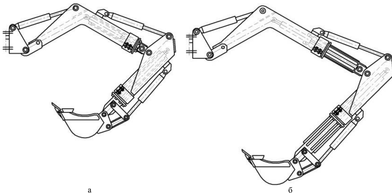
Рис. 11. Конструкція ТРО по а.с. України № 43969: а – телескопічне РО при втягнутих телескопах стріли та рукояті; б – ТРО при виштовхнутих телескопах стріли та рукояті..
