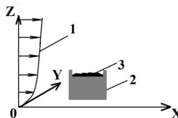
Рис. 2. Расчетная схема для 3D математического моделирования: 1 – профиль скорости ветра, 2 – полувагон, 3 – сыпучий груз / Sketch of 3D computational region: 1 – wind speed profile, 2 – wagon, 3 – bulk cargo
