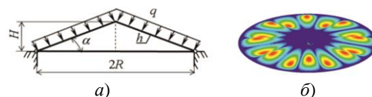
Рис. 3. Расчетная схема оболочки при шарнирном опирании основания (а) и форма потери устойчивости задачи 1 (б) / Loading schyme of the shell with hinged ends (a) and a buckling mode in problem no. 1 (b)
