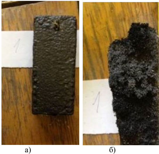
Рис. 1. Вид ВЗС, нанесеного на сосновый брусok розміром 60×30×150 мм: а) до випробувань; б) після випробування / Type of flame retardant intumescent composition applied to the pine block size of 60×30×150 mm: a) prior to testing; b) after the test
