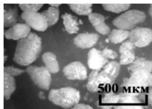
Рис.8. Структура вихідних алюмосилікатних мікросфер, просочених розчином TiO(SO_3CH_3)_2 \cdot nH_2O , після стадії прожарювання. / Structure of output aluminosilicate microspheres, impregnated with the solution TiO(SO_3CH_3)_2 \cdot nH_2O , after the firing stage.
