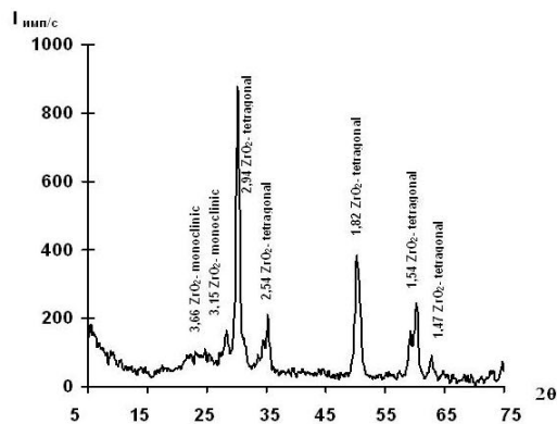
Рис.4. Рентгенівська дифрактограма алюмосилікатних сфер, просочених розчином ZrO(SO_3CH_3)_2 \cdot 4H_2O , після стадії прожарювання. / X-ray diffractogram of aluminosilicate spheres ZrO(SO_3CH_3)_2 \cdot 4H_2O , impregnated solution after the calcining.
