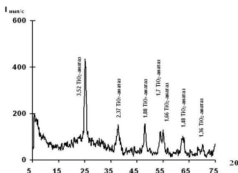
Рис.5. Рентгенівська дифрактограма алюмосилікатних сфер, просочених розчином TiO(SO_3CH_3)_2 \cdot nH_2O , після стадії прожарювання. / X-ray diffractogram of aluminosilicate spheres, impregnated with the solution TiO(SO_3CH_3)_2 \cdot nH_2O , after the firing stage.
