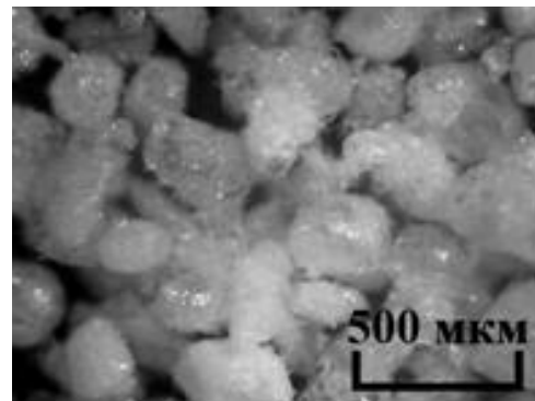
Рис.6. Структура вихідних алюмосилікатних мікросфер. / Structure of output aluminosilicate microspheres.
