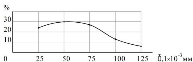
Рис. 5 График распределения частиц по крупности для порошков КСШ (кобальтовый сплав + шпинель), \delta – размер частиц в мкм. / Fig.5. Graph of particle size distribution for spinel powders CAS (cobalt alloy+spinel) \delta – partical size in mkm.
